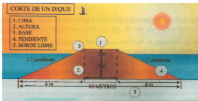
Figura 10. Esquematización del dique de un estanque (Tomada de Ramírez, 2003).
