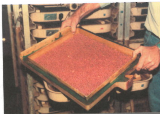
Figura 27. Incubadoras para huevos y larvas de trucha arco iris y salmón.
